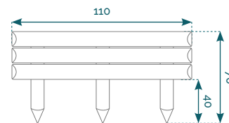
BOPLDR-70x40-110
