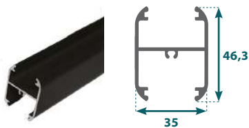
Traverse intermédiaire
