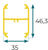
Traverse intermédiaire
