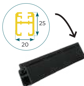
Profil d'encadrement
