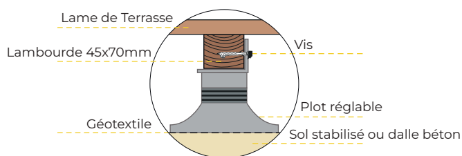
POSE SUR PLOTS
