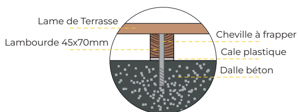
POSE SUR DALLE BÉTON
